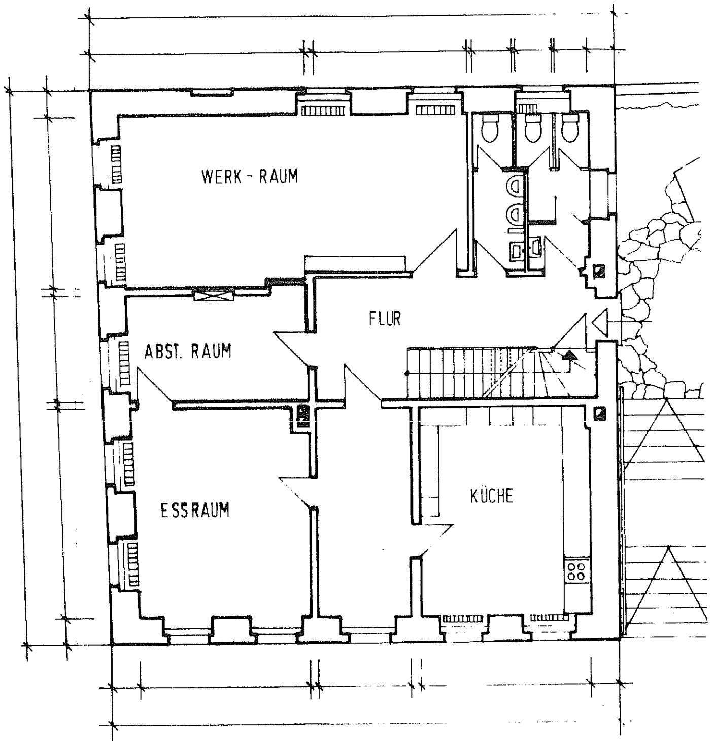
ERDGESCHOSS
